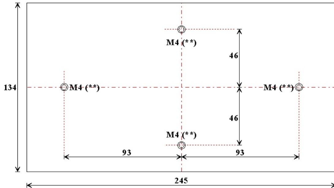
VISTA DA SOTTO / BOTTOM VIEW
